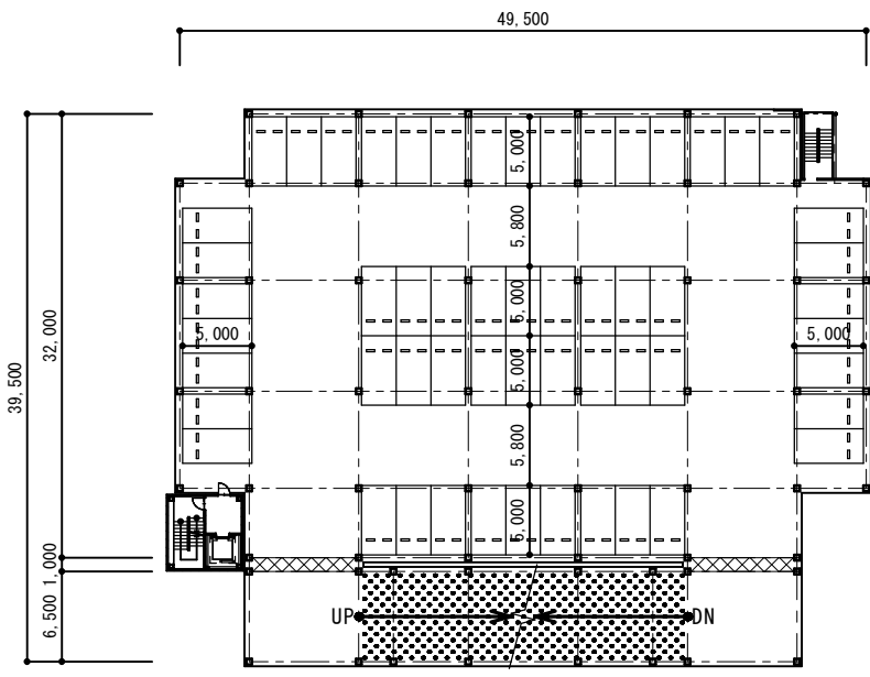
2～6階平面図
