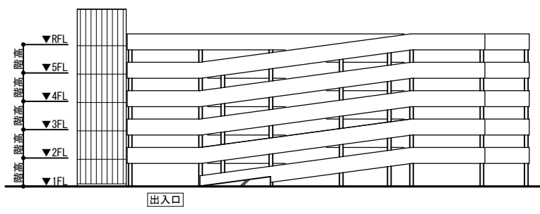
立面図
