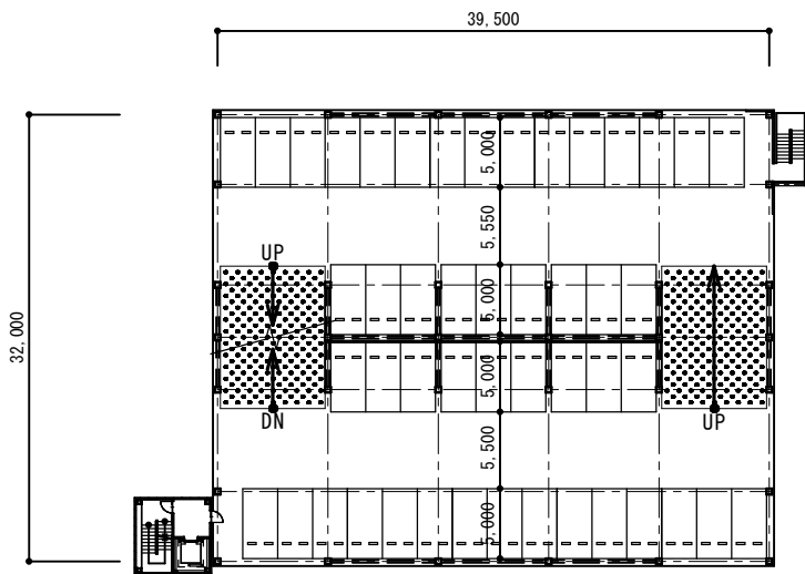
2~5階平面図
