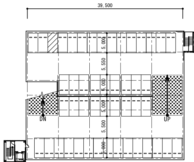
R階平面図
