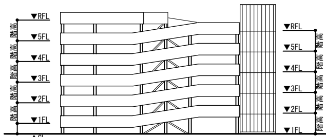
立面図
