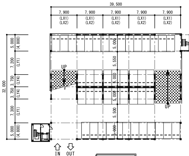
1階平面図
