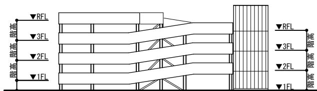
立面図
