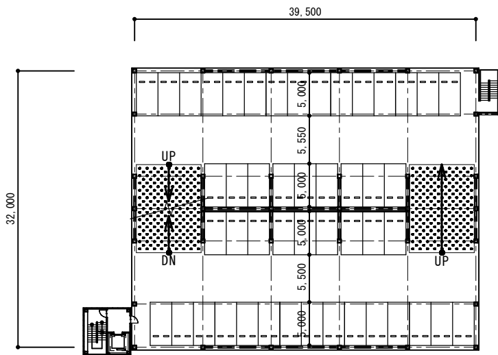
2・3階平面図
