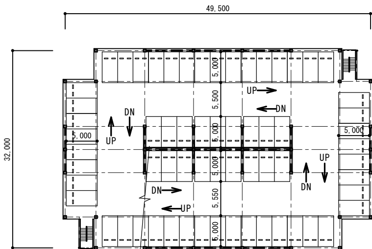
2階平面図
