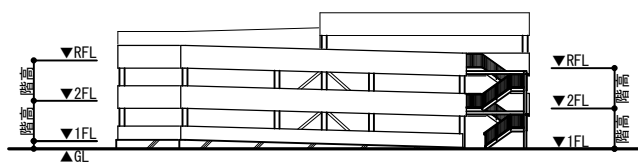
立面図
