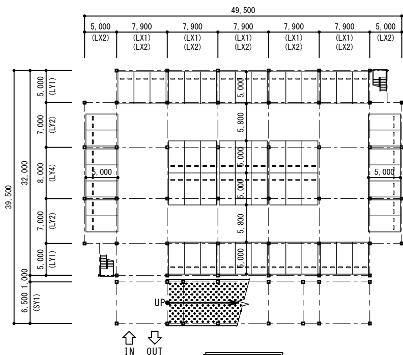
1階平面図
