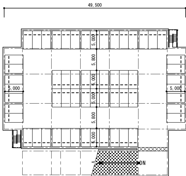
R階平面図
