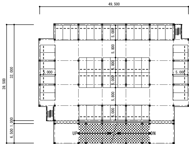
2階平面図
