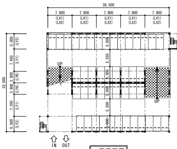
1階平面図
