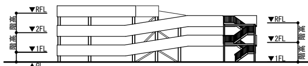
立面図
