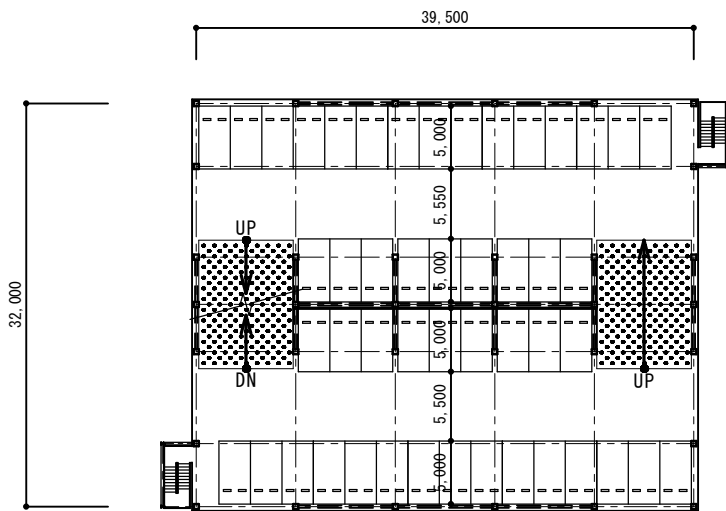
2階平面図
